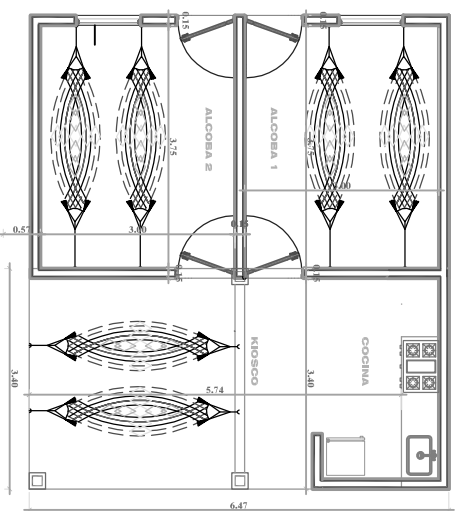
PLANO ARQUITECTONICO
